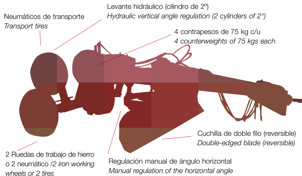
Terrena Big 8442 con rueda de hierro, with Steel wheels
